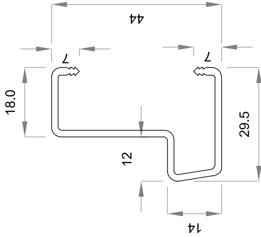
OPDEKDEURPROFIEL
